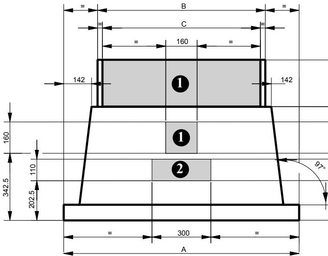
RÜCKANSICHT
