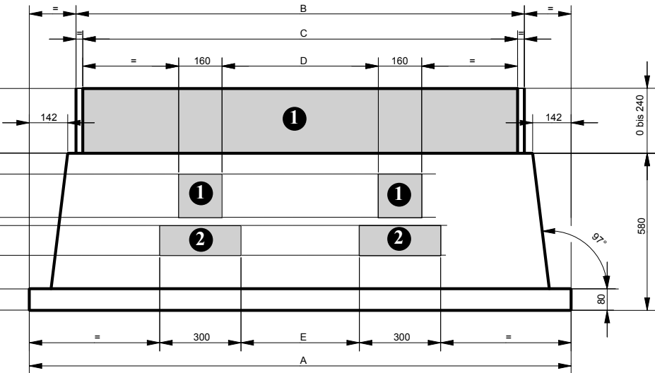
RÜCKANSICHT
